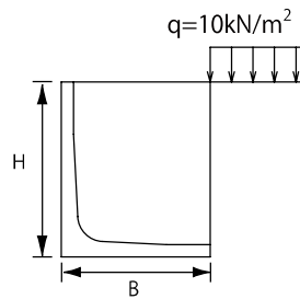
ケース2 自重 + 土圧
