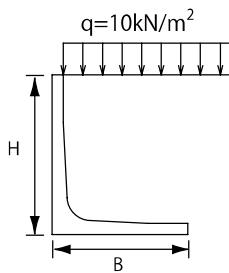
ケース1 自重 + 載荷重 + 土圧
