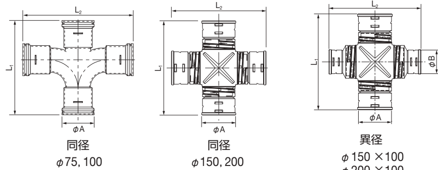
異径 単位: mm
