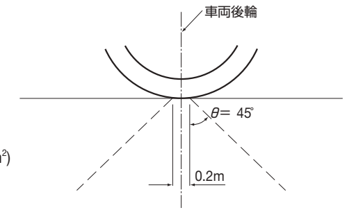
輪荷重の分布
