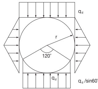
(a)鉛直荷重による土圧分布
