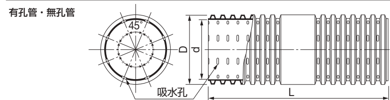
トヨドレンダブル管製品構造図
