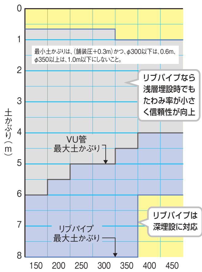
リブパイプとVU管の適用土かぶり
