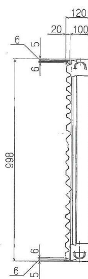
法砂ブロック ～新タイプ～ 製品図
