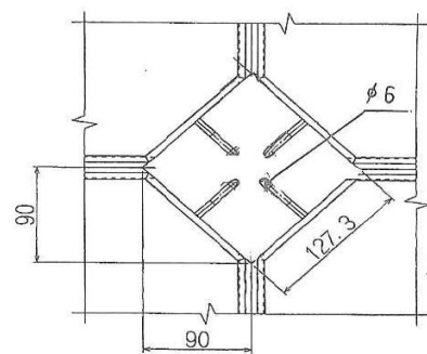
施工時 連結部
